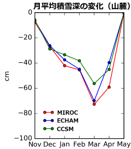
図1 アンヌプリ山山麓における現在気候に対する月平均積雪深の将来変化。
