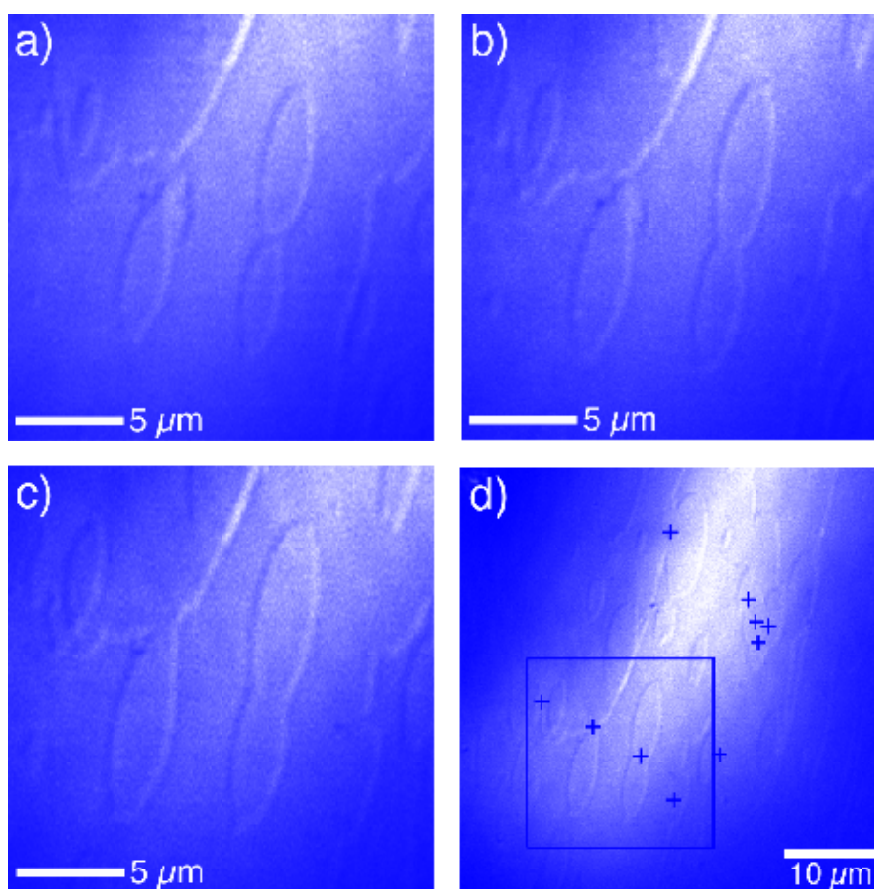
図5 レーザー共焦点微分干渉顕微鏡を用いてその場観察した、鶏卵白リゾチーム正方形系結晶{110}面上での2次元核成長. ステップの高さ：5.6nm. (a) 0 秒, (b)26.9 秒, (c),(d)53.8 秒. (d)において、図中の四角は(a)-(c)で観察している領域を、そして+印は隣り合った2次元島の合体に伴い、ステップのコントラストが消滅した部位を示す.
