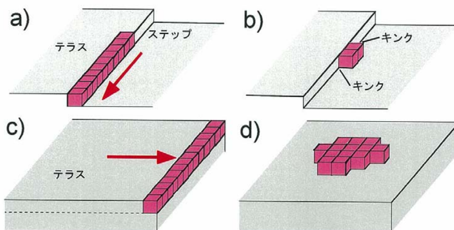
図4 結晶の沿面成長メカニズム. a)ステップに沿ったキンクの成長. b)ステップ上での1次元核形成(2つのキンクが新たに生成). c)ステップが結晶端まで成長. d)テラス上での2次元核形成.
