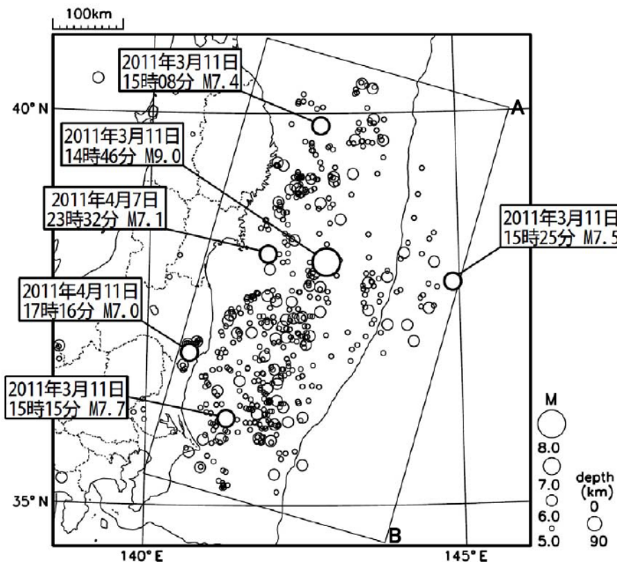
図3 「平成 23 年（2011 年）東北地方太平洋沖地震」の地震活動 2011 年 3 月 11 日 12 時～2011 年 6 月 8 日 08 時までに発生した地震(M \geq 5.0、深さ 90km 以浅)の「平成 23 年(2011 年)東北地方太平洋沖地震」の震央分布図。○の大きさはマグニチュードを表す。吹き出しは M7.0 以上の地震に付けた。
