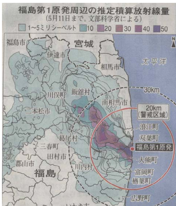
図8 福島第1原発周辺の推定積算放射線量 (3月11日～5月11日)
