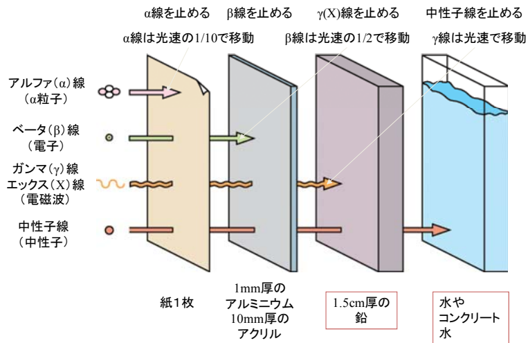
図5 放射線の種類と透過力
